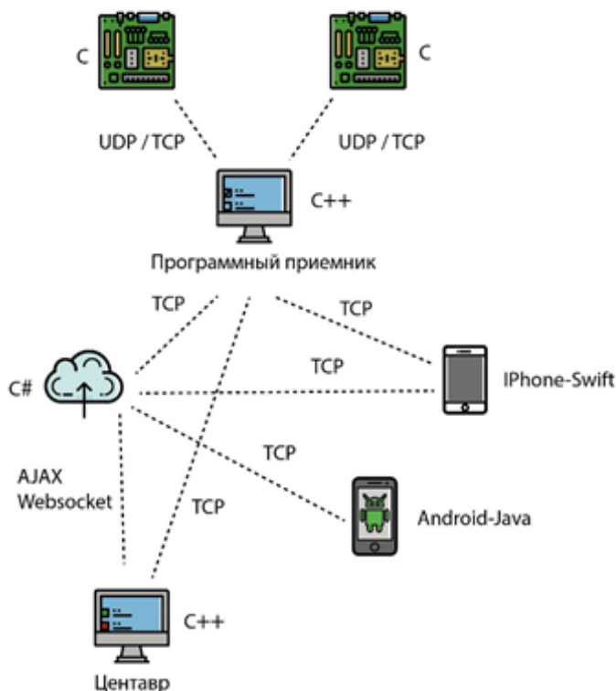
Рис 1. Структурная схема
